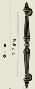
Maniglione Colosseo Bronzo Yester MT160.R8.BY Colosseo Yester Bronze pull handle
