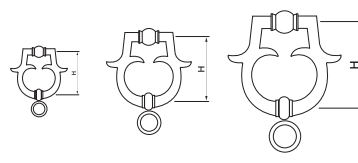
Art. 10B H. 120 mm ART. 10A H. 150 mm ART. 10G H. 180 mm
